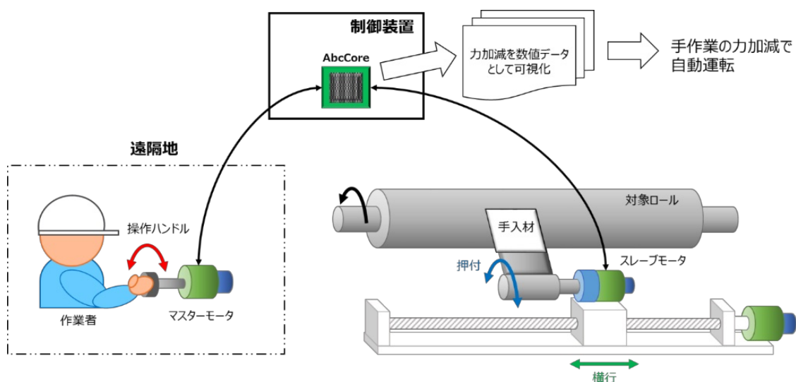
図1 開発システムの概要図
